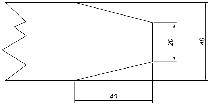
Detalle extremos platabandas en consolas
