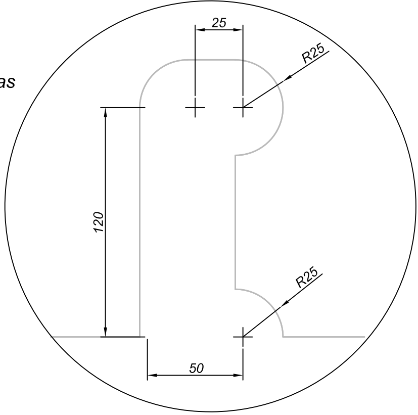
Detalle extremos platabandas en consolas
